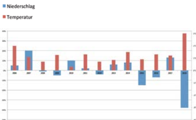
Temperatur- und Niederschlagsabweichung von langjährigen Mittel in den Jahren 2006 bis 2018
